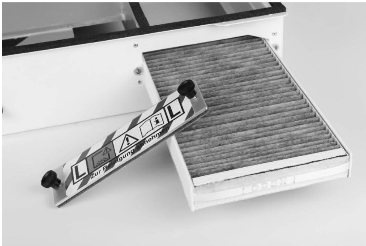
Photo # 2 -. Unité l'élément de filtre principal retiré ainsi que l'ouverture pour le changement de filtre.
